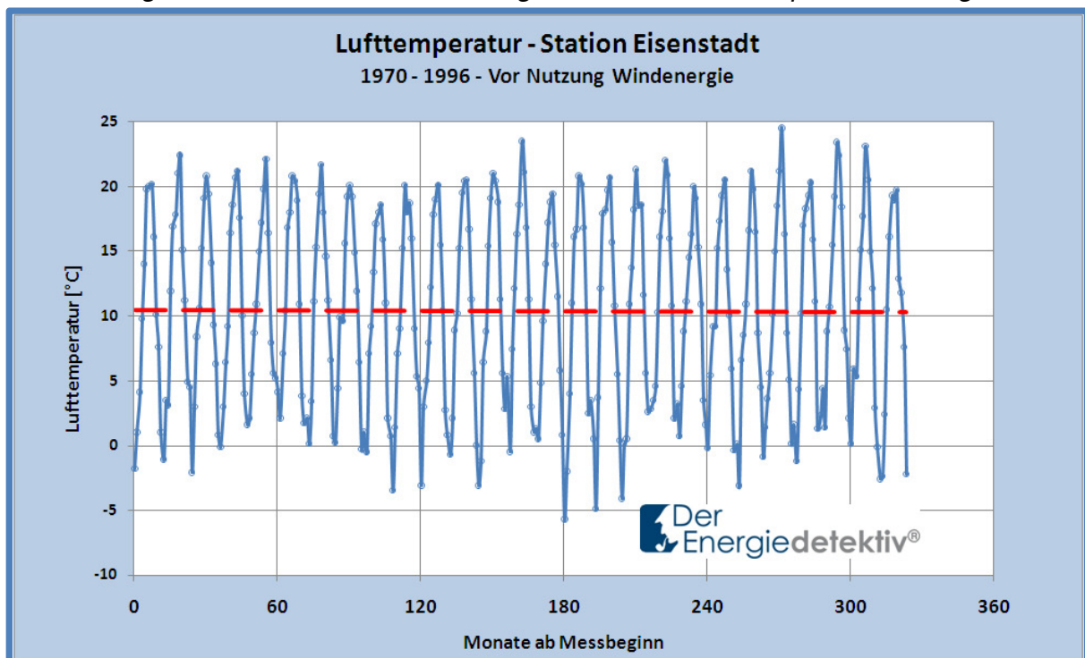
Bild 5: Temperaturverlauf für den Zeitraum 1970 bis 1996. Diese gleich lange Zeitperiode vor Nutzung der Windkraft zeigt keine Trendänderung.
