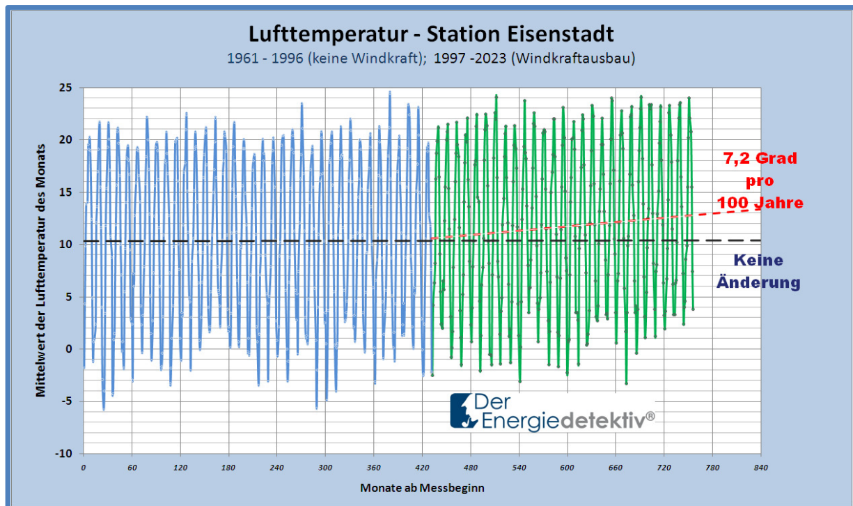
Bild 3: Temperaturverlauf seit 1961; die blaue Kurve entspricht der Zeit ohne Nutzung der Windkraft. Die grüne Kurve zeigt den Verlauf ab Nutzung der Windenergie. Die Veränderung im linearen Trend ist höchst alarmierend!
